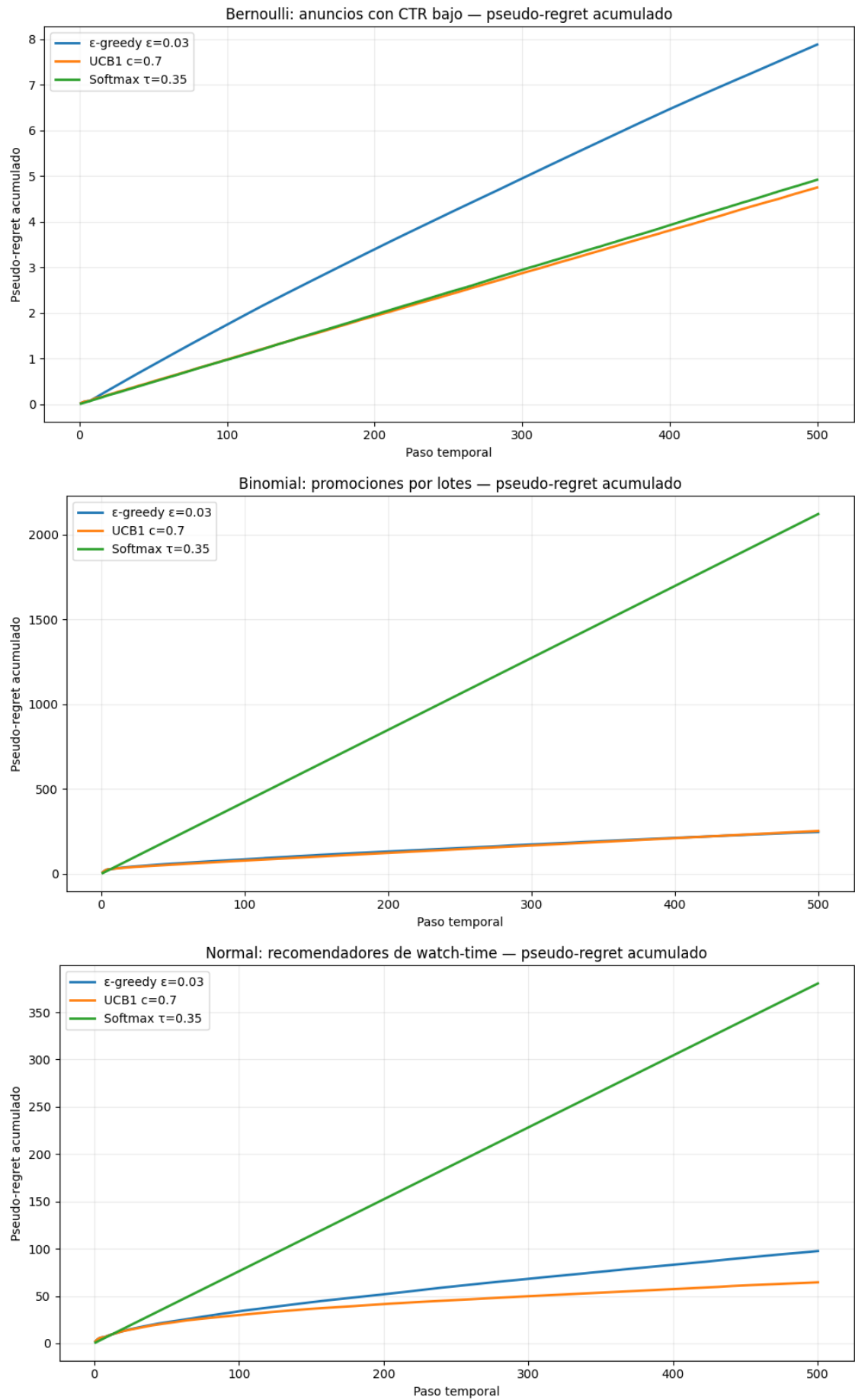
Figura 1: Ejemplo de curva de pseudo-regret acumulado para la comparación transversal.
